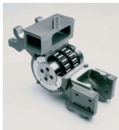
Цилиндрические роликоподшипники с полиамидным сепаратором
