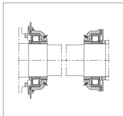
Моторно-осевая подшипниковая опора – цилиндрические роликоподшипники
