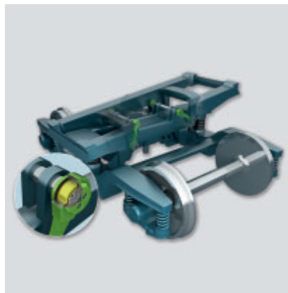
Главная тележка вагона
