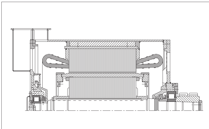
Тяговый двигатель
