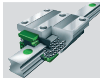
Четырёхрядная линейная направляющая качества с циркуляцией шариков KUVE..-B
