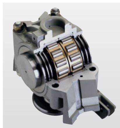
Цилиндрические роликоподшипники с латунным сепаратором для внутренней опоры
