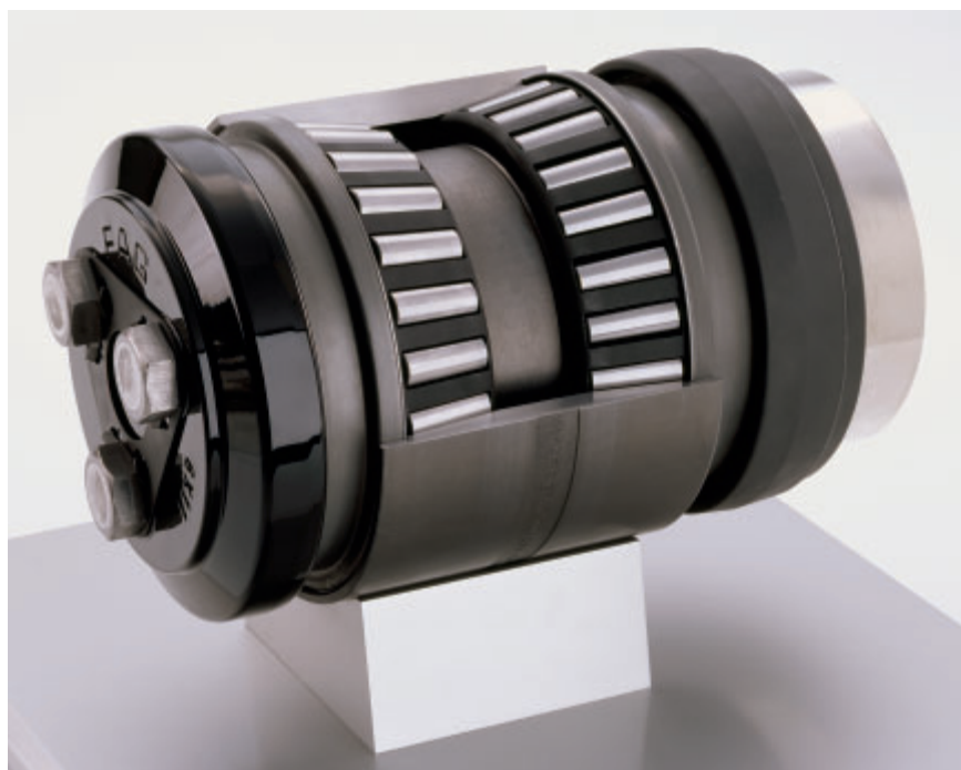
Вид узла TAROL с размерами в дюймах
